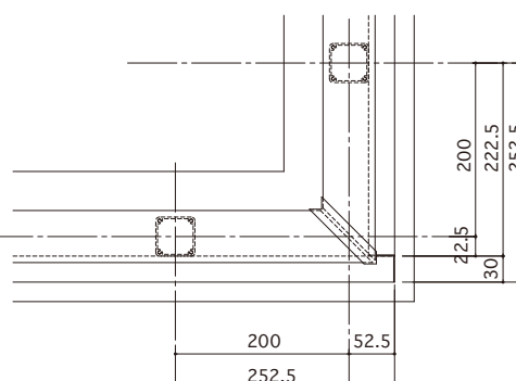
出隅コーナー部納まり
