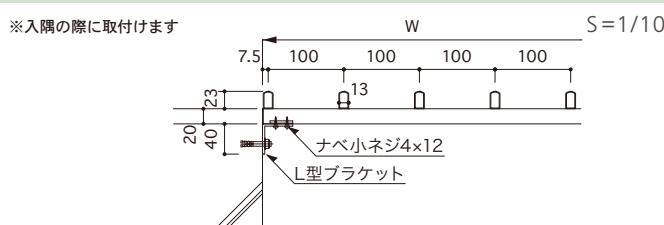
納まり L型 ブラケット
