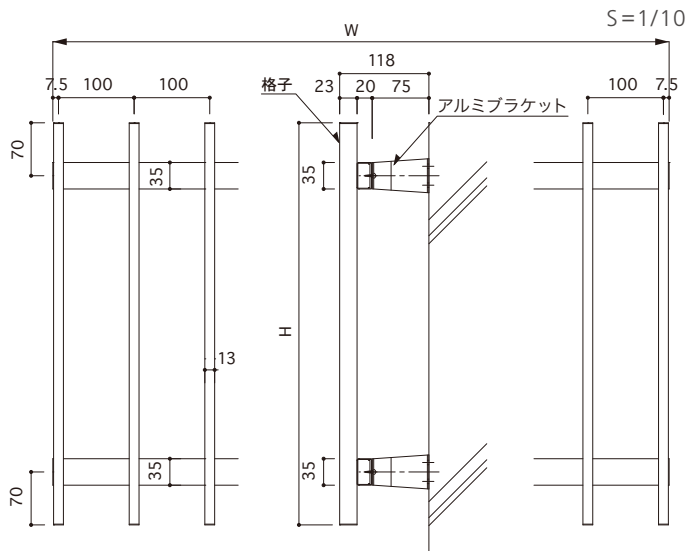
納まり ドア用面格子
