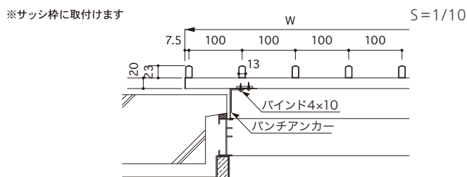
納まり L型 ブラケット
