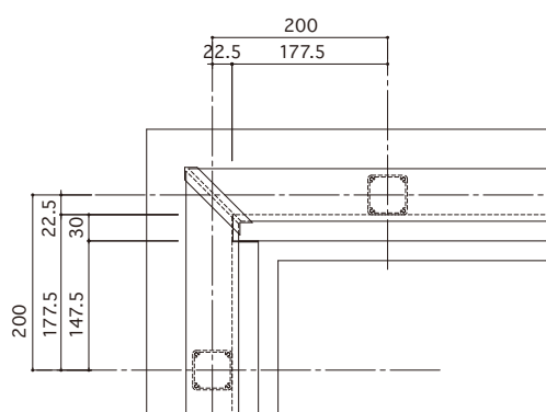
入隅コーナー部納まり
