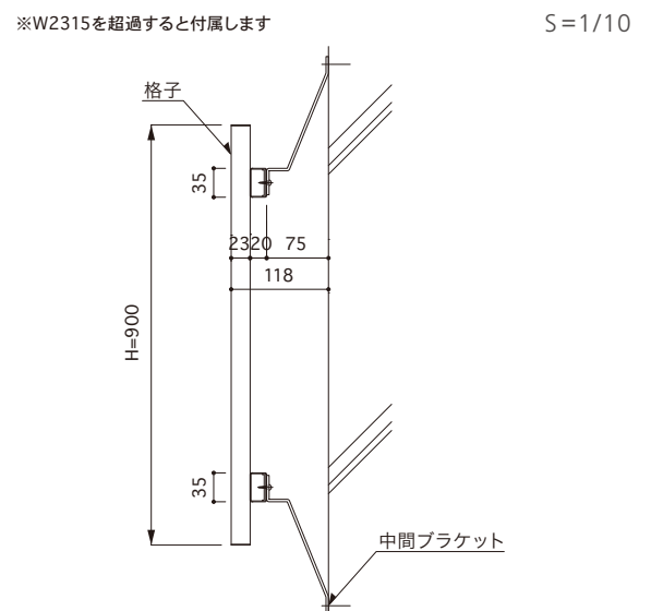
納まり 中間ブラケット
