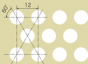
丸孔千鳥タイプ E 開口寸法：8φ×12P 開口率：40%
