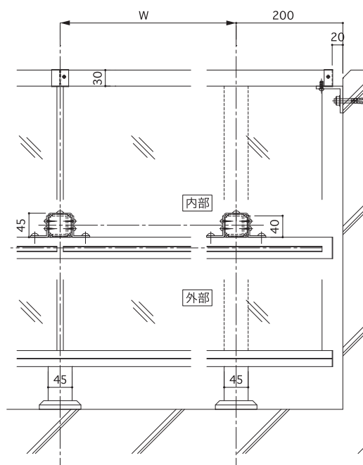
端部堅枠なしの場合
