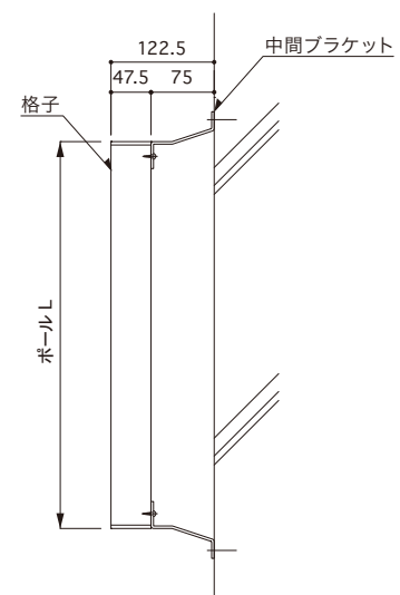
納まり 中間ブラケット
