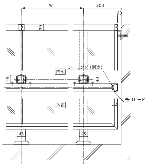
端部堅枠ありの場合 シーリングなし
