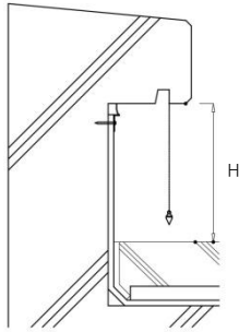
T-1工法
