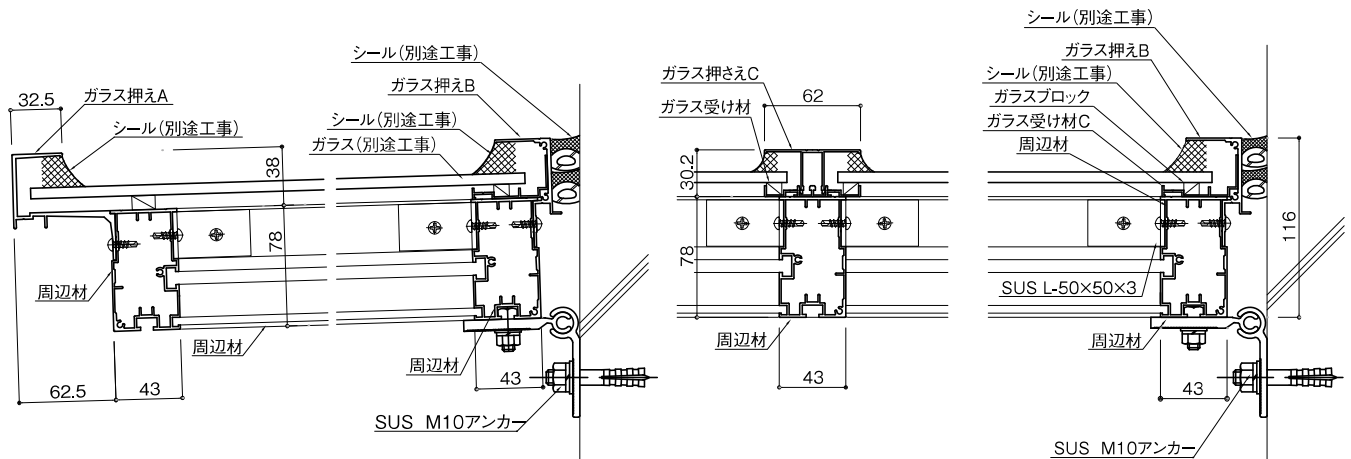
水 下 軒先部
