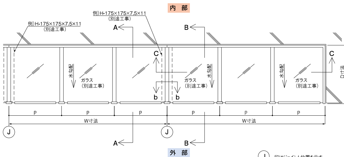
底平面図
