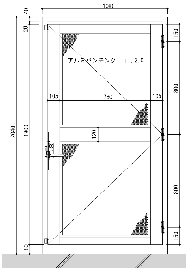
非常用(破壊錠)格子扉
