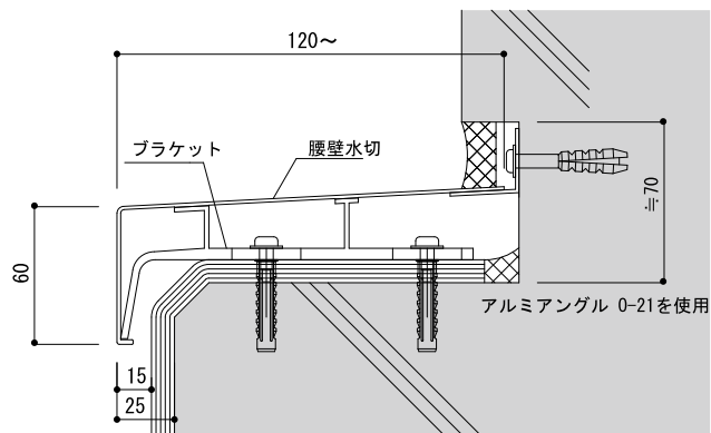
オプション水切 OH-45F
