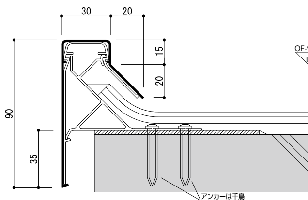
OF-90E(シルバーのみ) L=2000
