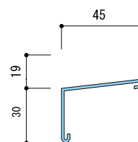
オプション水切 OH-45F
