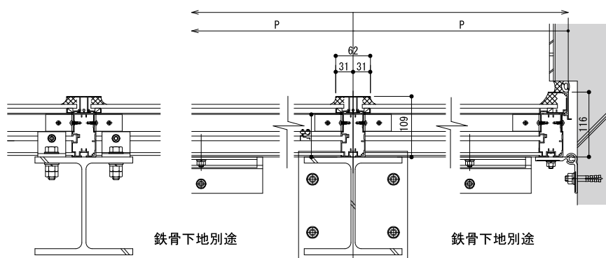
C-C 断面图
