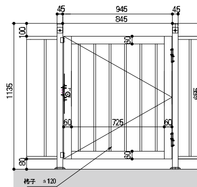
非常用(破壊錠)格子扉
