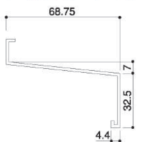
ボード用水切ジョイント材
