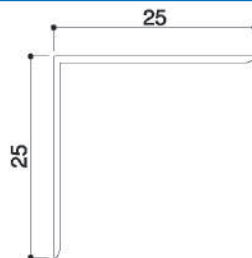
コーナーアングル
