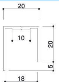
上部レール
