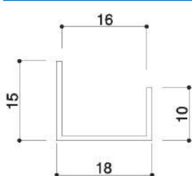
下部レール
