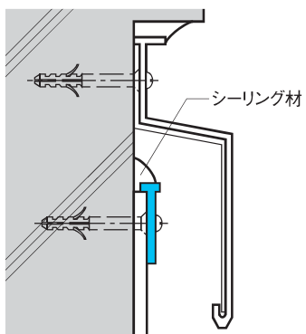
(水切・アングル納まり図)
