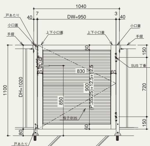
——片開き門扉——
