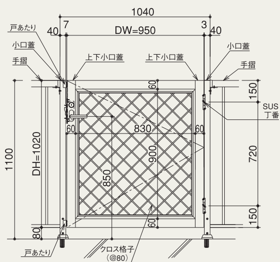
—— 片開き門扉 ——
