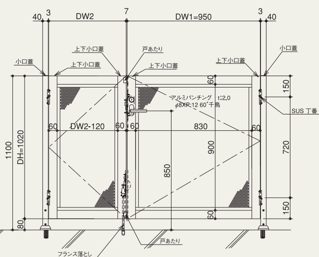
—— 親子門扉 ——
