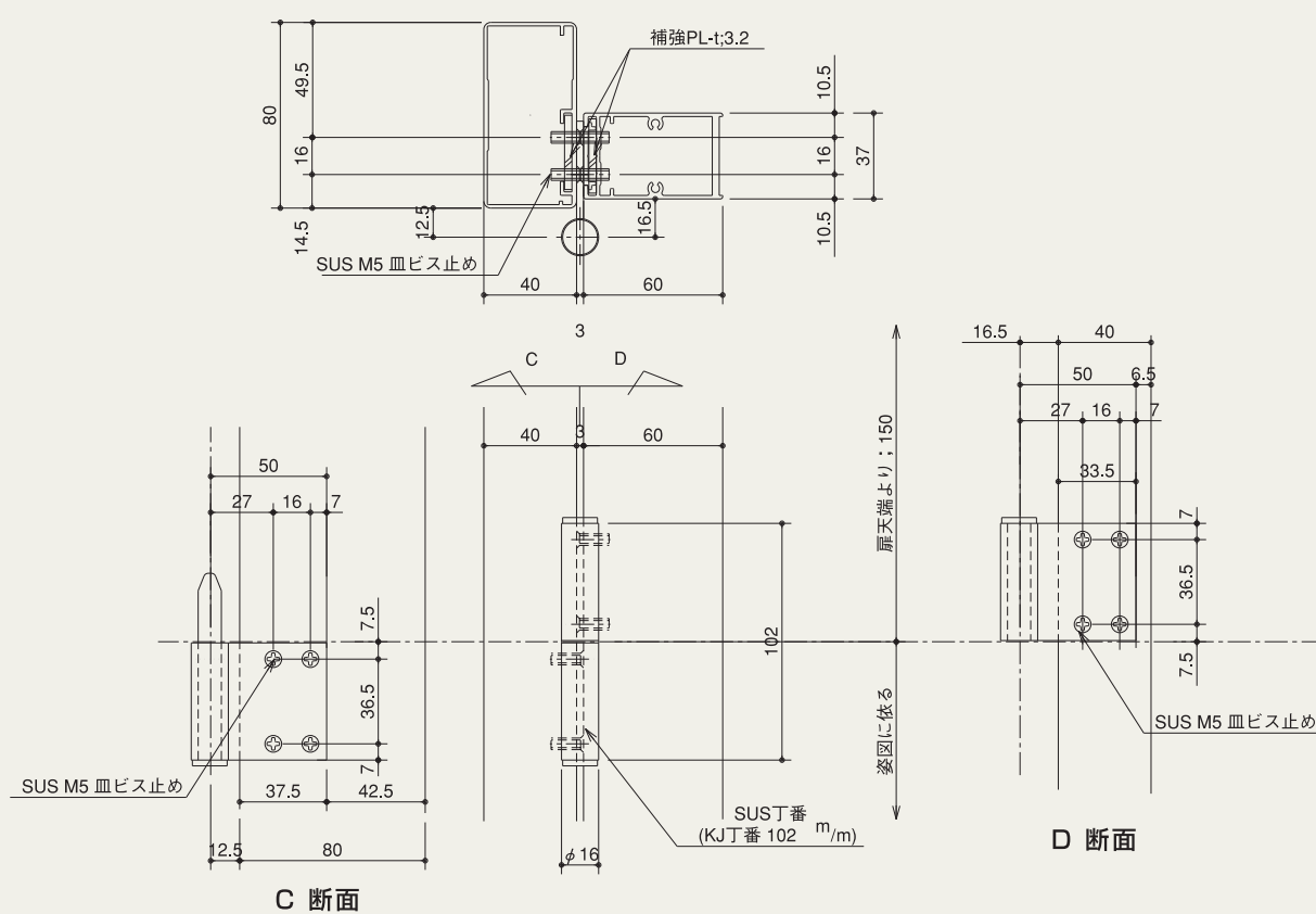
丁番部 詳細図
