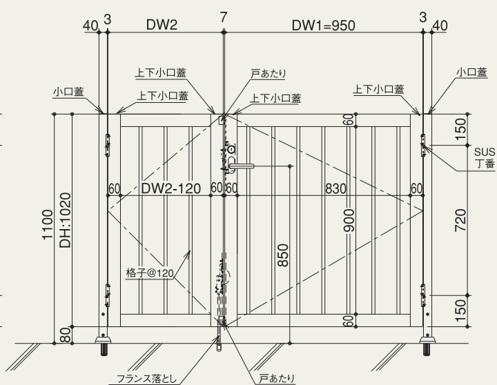
—— 親子門扉 ——
