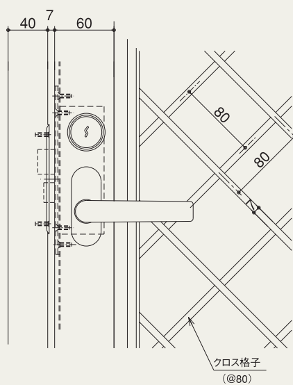
鍵詳細図
