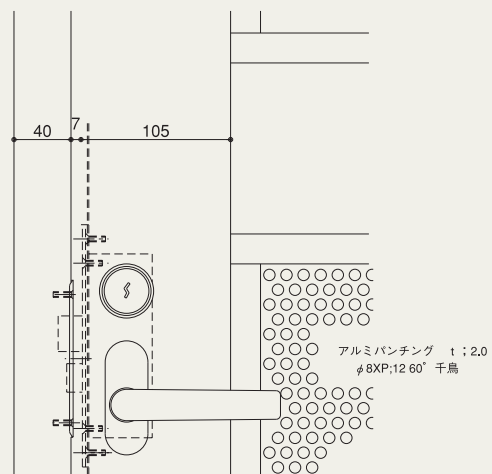
鍵詳細図
