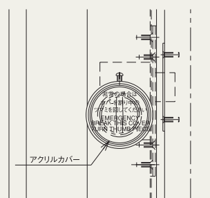
内部側鍵立面図
