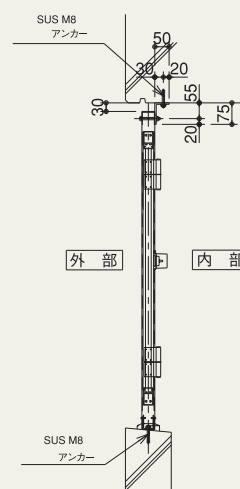
断面図
