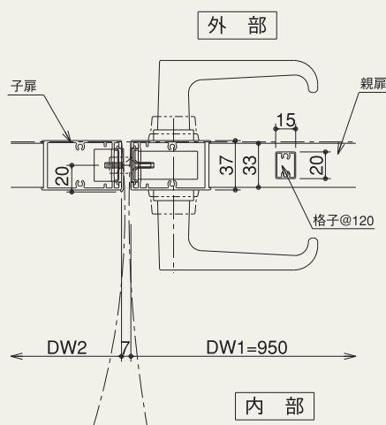
平断面詳細
