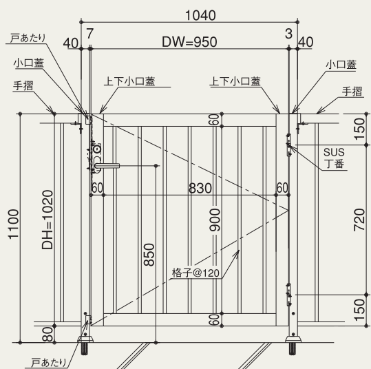
——片開き門扉——
