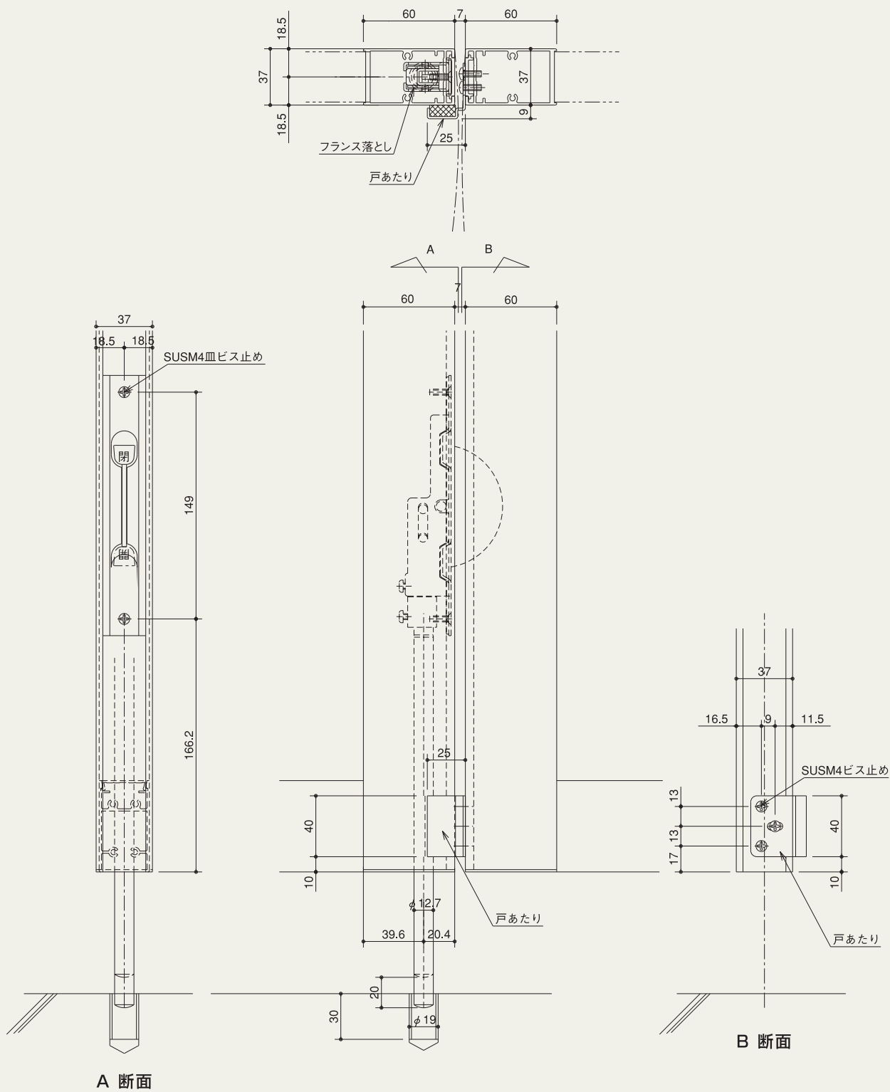
フランス落とし、戸あたり詳細図
