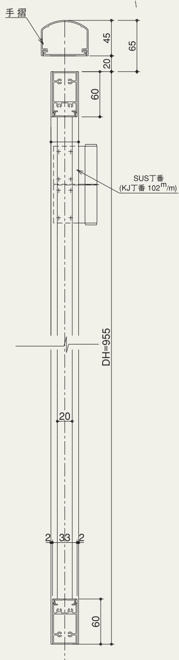
立断面詳細
