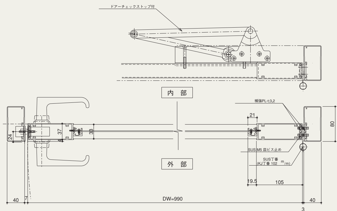
平断面詳細
