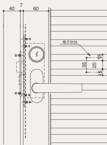
鍵詳細図
