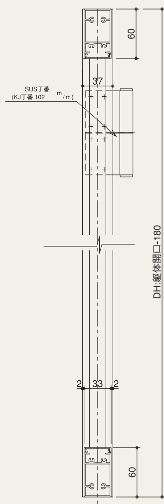
立断面詳細
