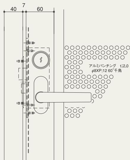
鍵詳細図
