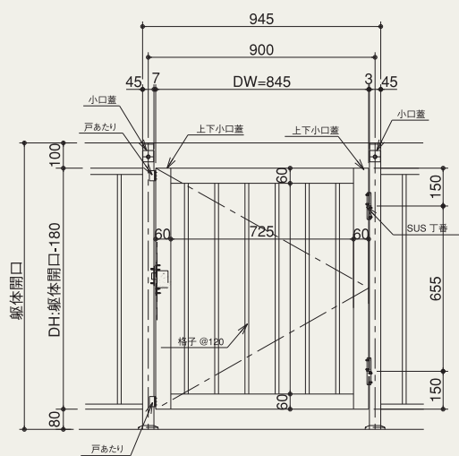
立面図
