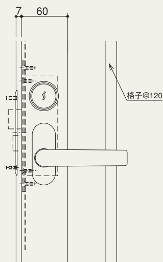
鍵詳細図
