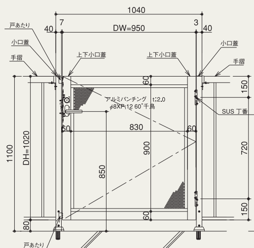
—— 片開き門扉 ——
