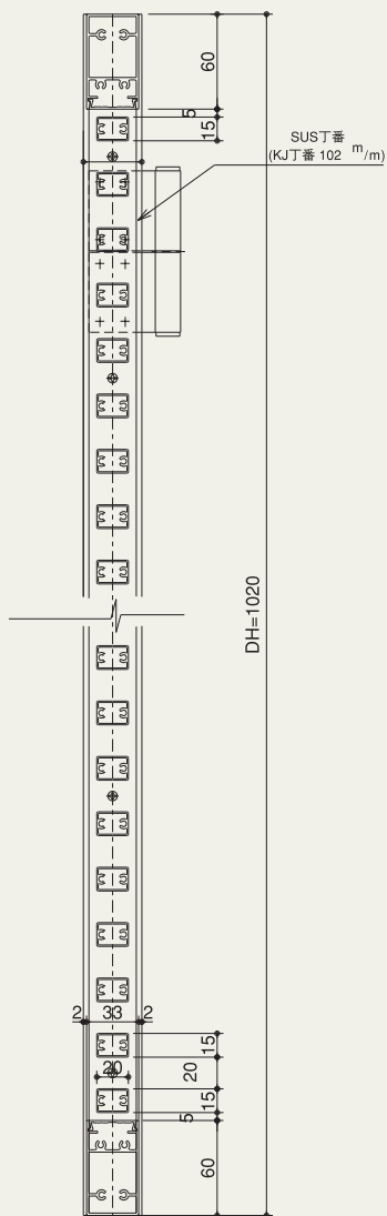
立断面詳細
