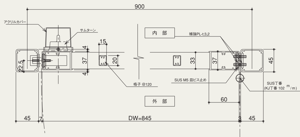
平断面詳細
