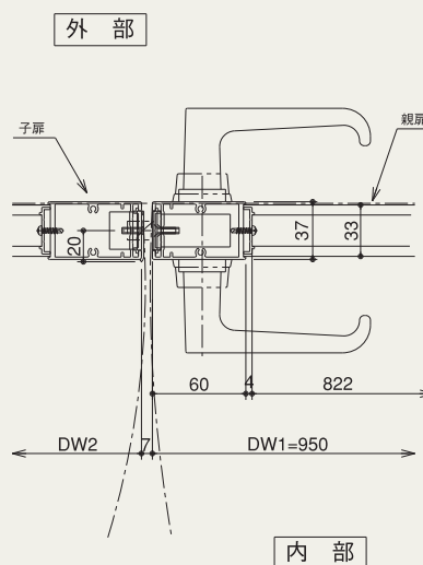
平断面詳細
