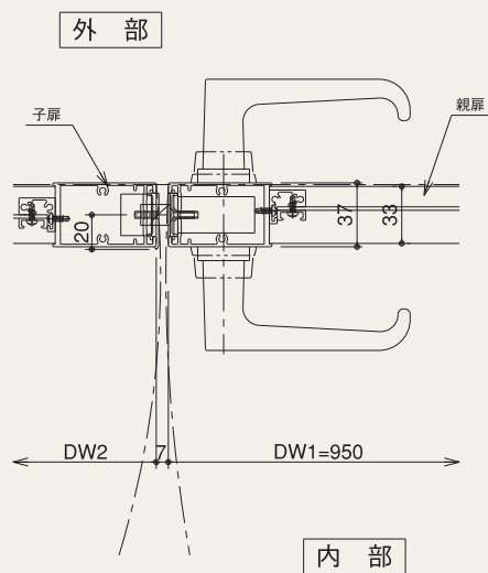
平断面詳細
