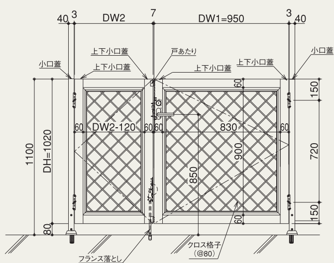
—— 親子門扉 ——
