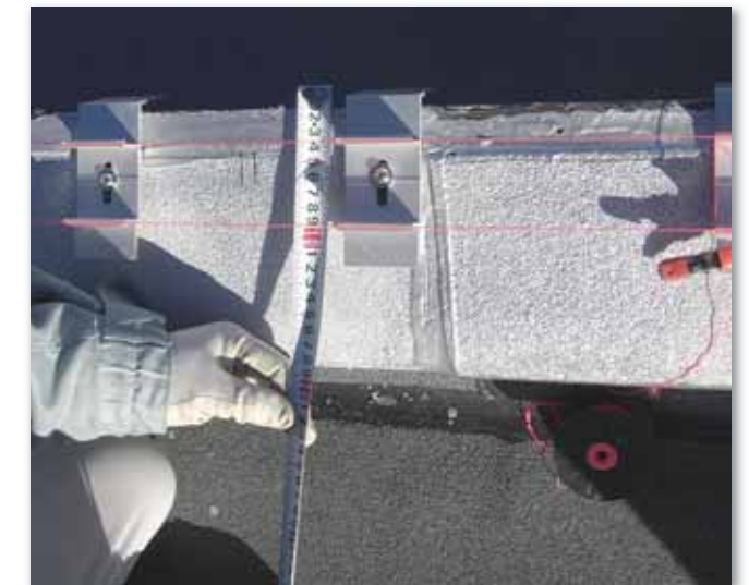
改修中（半笠木+むね上げ導体対応）
