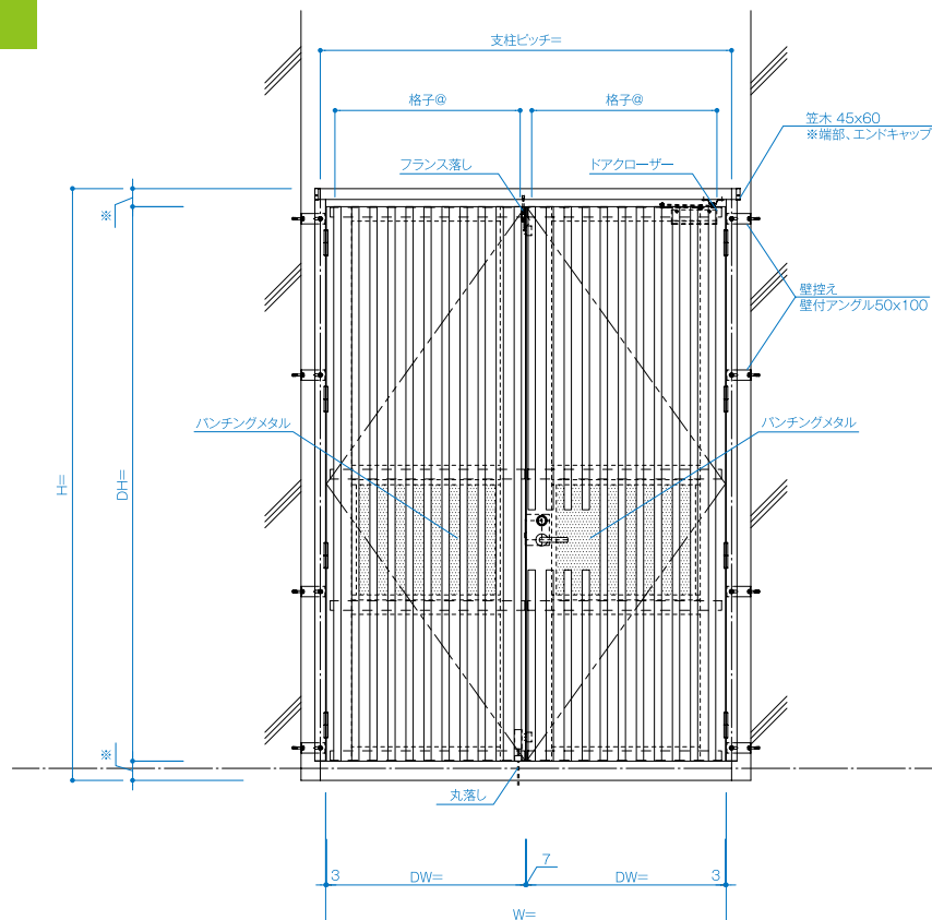
立面図
