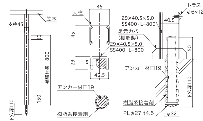
支柱補強材 HBK-38C 手すり笠木ブラケット HBK-41C
