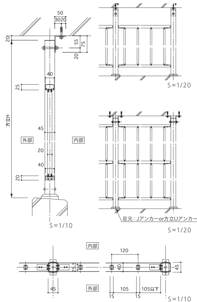
納まり 侵入防止柵
