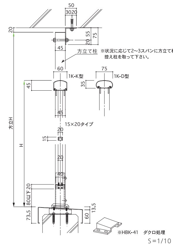
納まり 手すり付笠木
