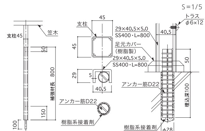
支柱補強材 HBK-30A
