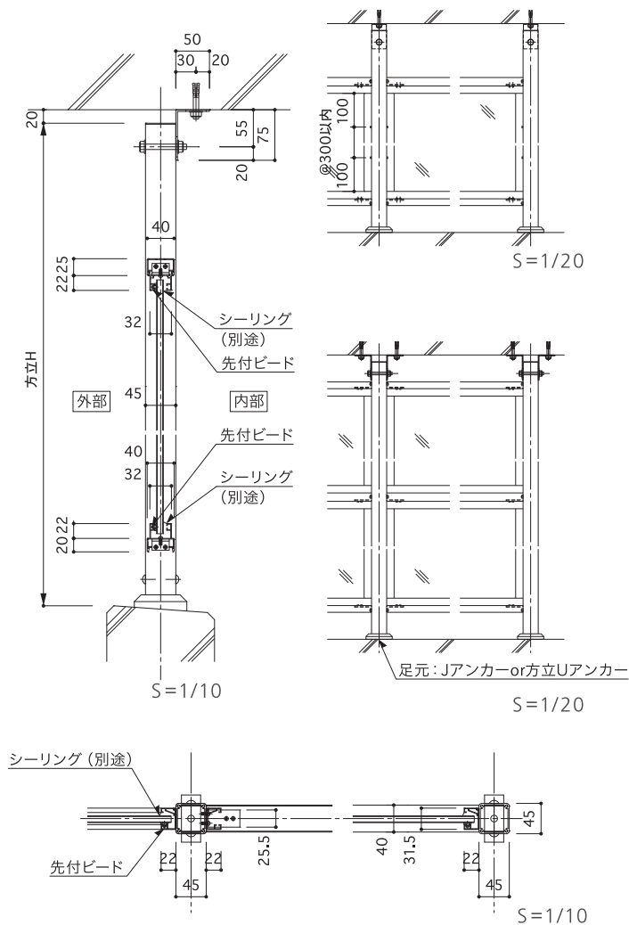
納まり 目隠スクリーン
