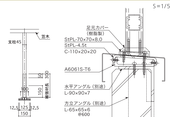
支柱補強材 HBK-38C 手すり笠木ブラケット HBK-41C
